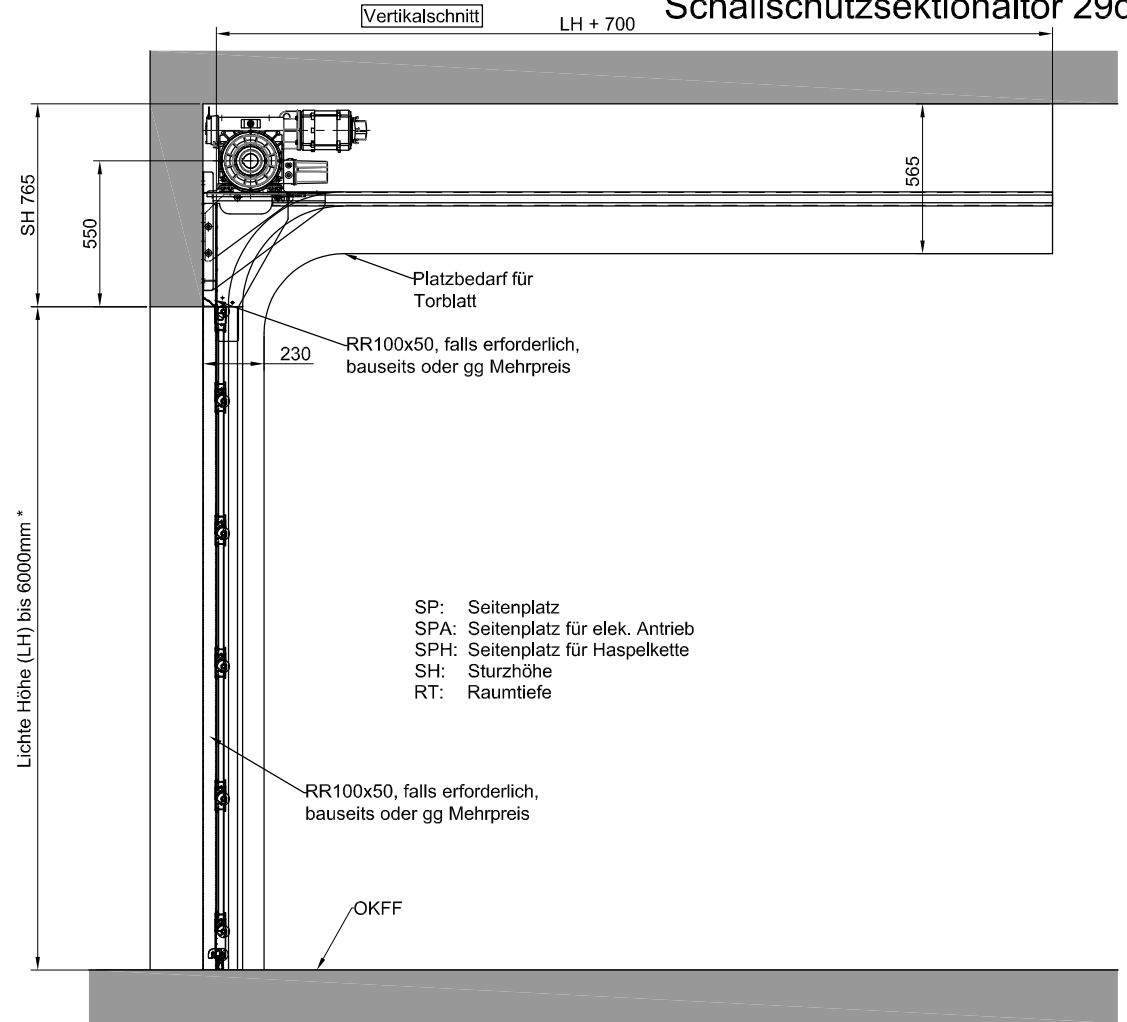
Vertikalschnitt
