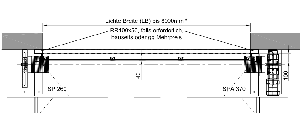
Horizontalschnitt
