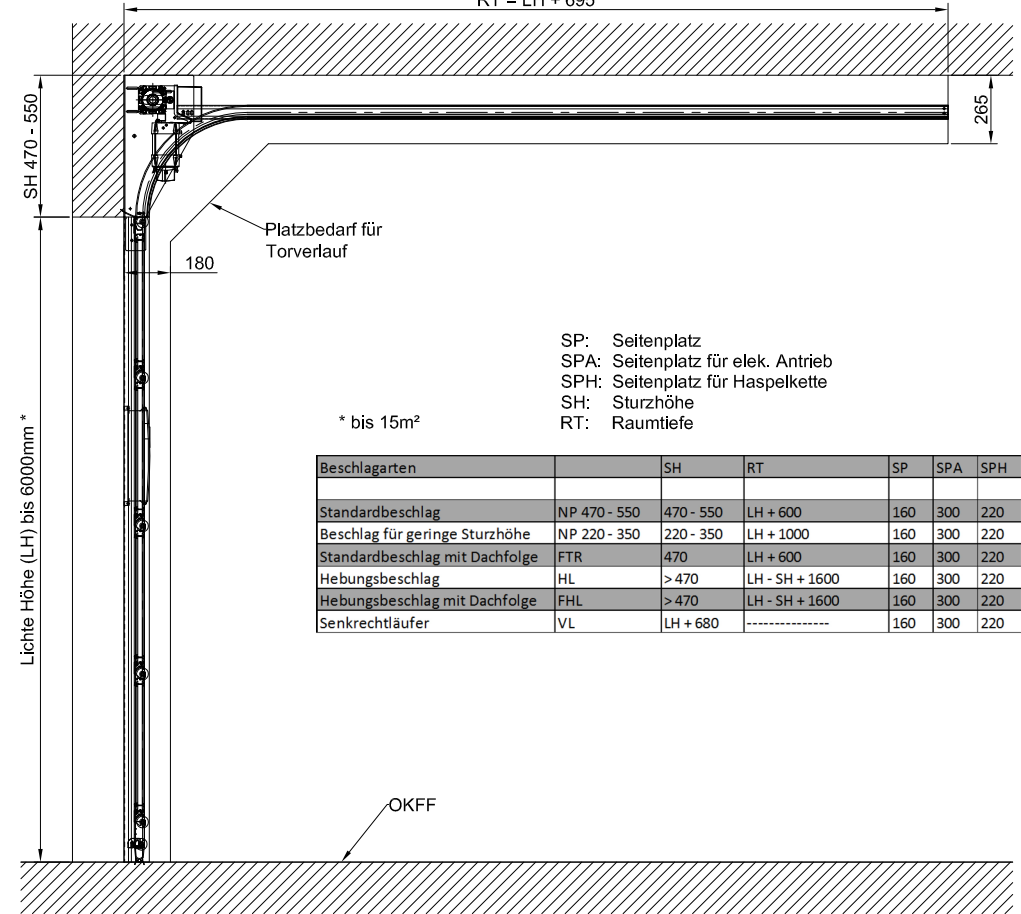
Vertikalschnitt
