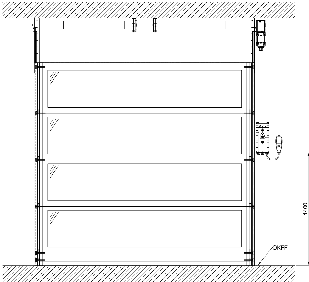
Gesamtansicht Innen
