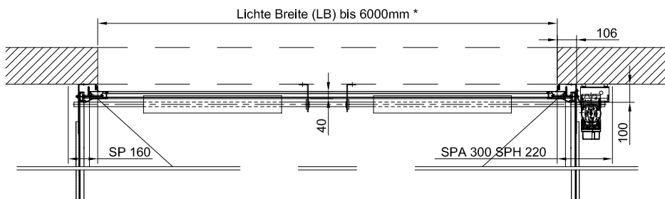
Horizontalschnitt
