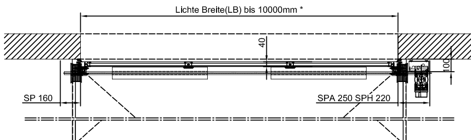
Horizontalschnitt
