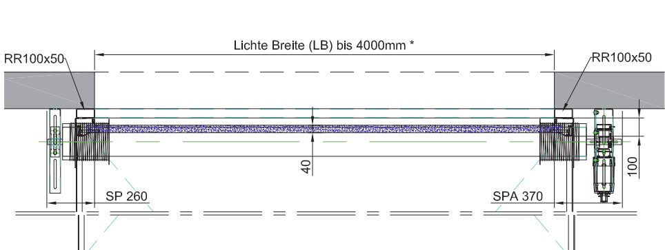
Horizontalschnitt
