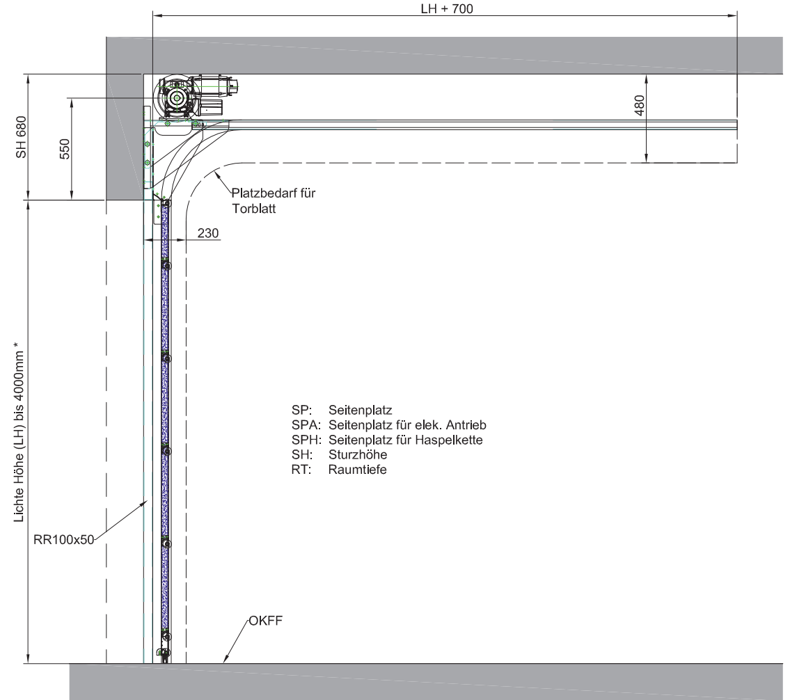
Vertikalschnitt
